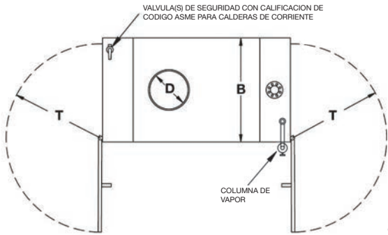
VISTA DE ARRIBA ④
