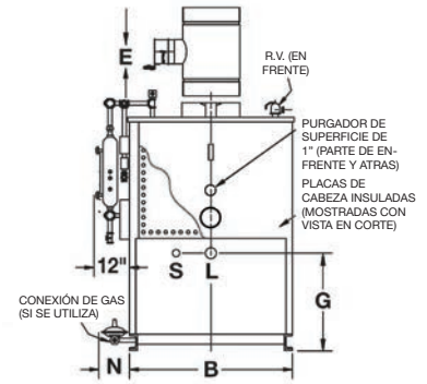
VISTA DE ATRÁS ④
